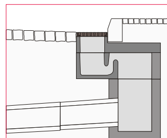
Caixa de Sarjeta de 60 ou Caixa de Sarjeta de 80
