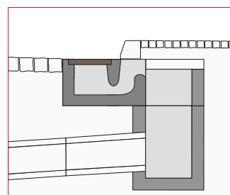
Caixa de Sarjeta de 60 ou Caixa de Sarjeta de 80
