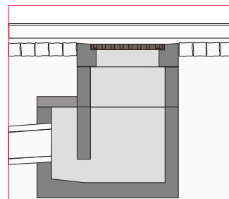
Acrescento de caixa
