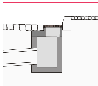
Caixa de Sarjeta de 60
