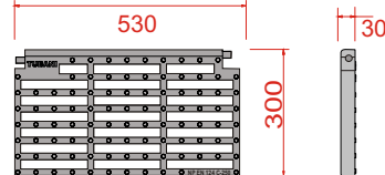
Alçado do aro da Grelha
